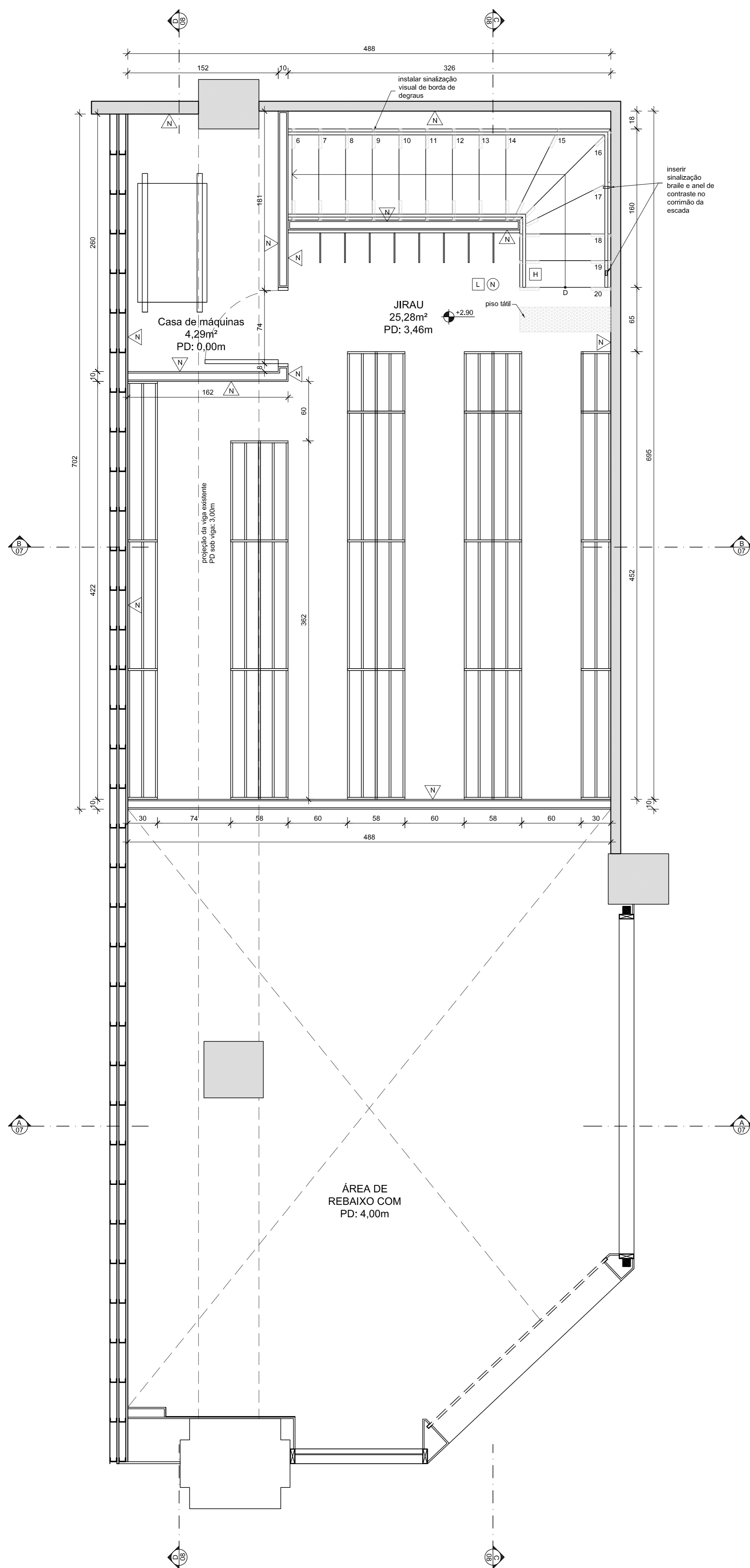
1 Planta baixa ESCALA: 1:25
