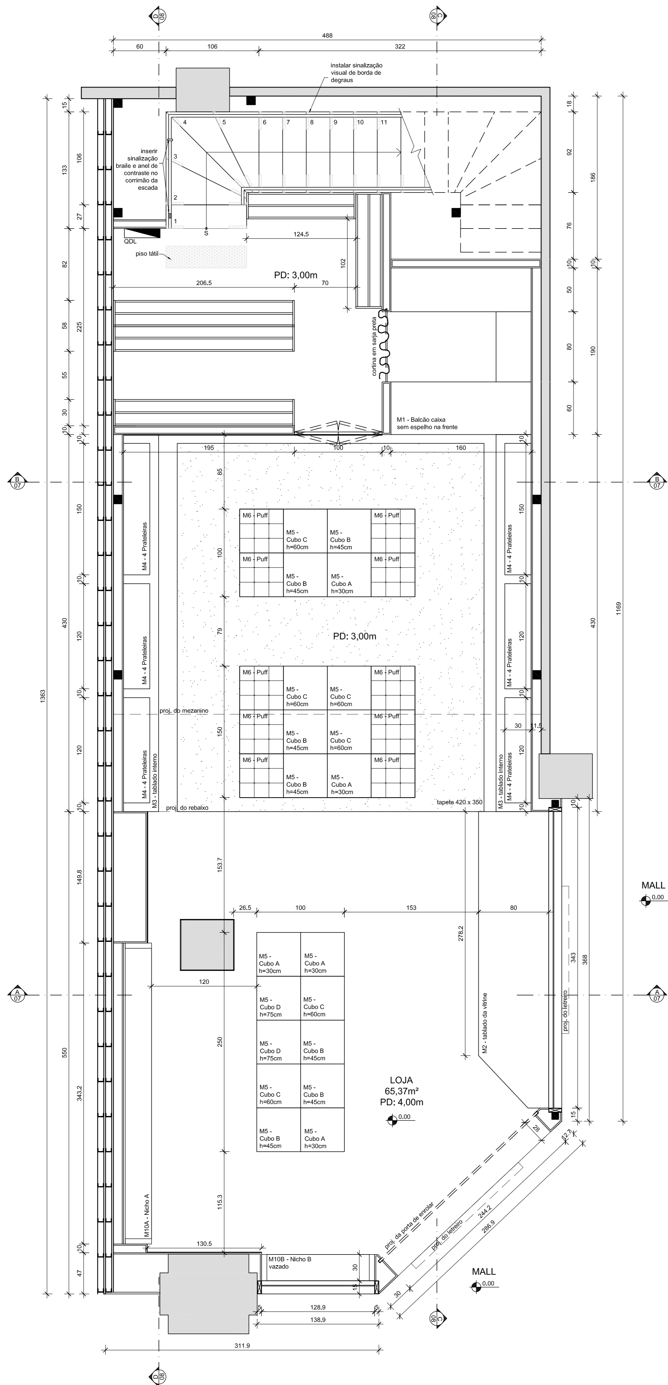
1 Planta baixa - layout ESCALA: 1:25
