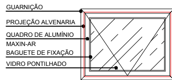
JA80 - VISTA INTERNA S/ESC.
