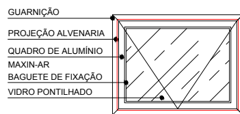
JA80 - VISTA INTERNA ESCALA 1:25
