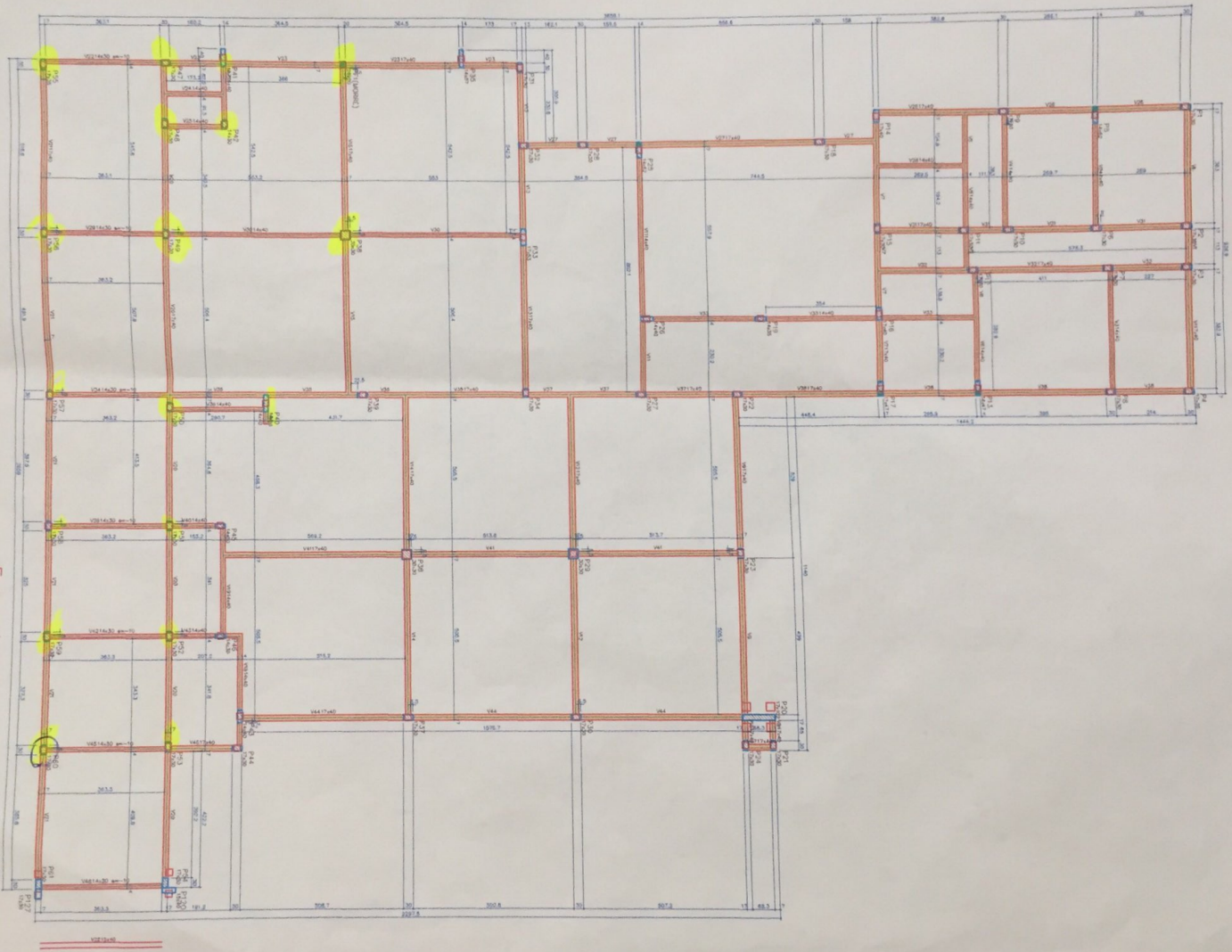
Forma do pavimento Baldrame (Nível 0) escala 1:50
